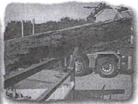
Links: Potbalk, rechts draagbalk van de kruissteiger (Foto: Joep Gründemann)
