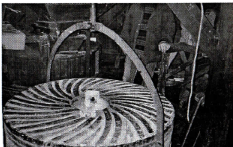
ter hoogte van de rand van de potjes in de steen bevindt zich een "ring", een verhoging van zo'n 3 mm, terwijl de buitenomtrek een 'verlaging' heeft, dit heeft dus als gevolg dat de stenen niet goed kunnen malen G. Ijpmā
