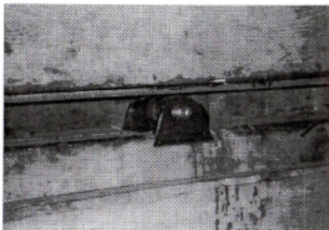
het aparte "engels kruiwerk" van de Sint Nicolaasmolen in Denekamp waarbij alleen de neuten zijn vervangen door rollen, ditzelfde geldt voor de keerkuip
