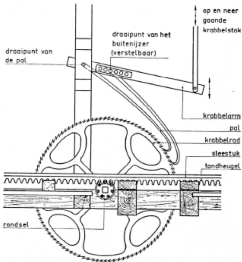
Het krabbelwerk van een zaagmolen. (Naar Boorsma)
